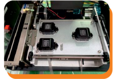
Cap İstasyonu
